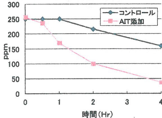
メチルメルカプタンガス推移
