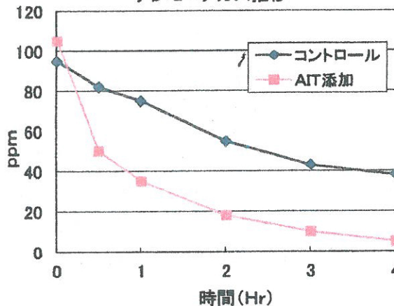
アンモニアガス推移
