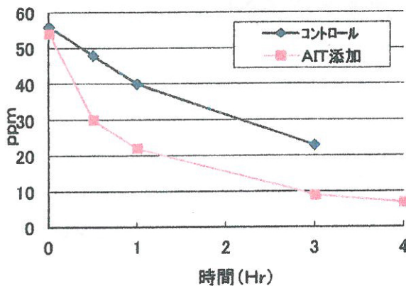
硫化水素ガス推移
