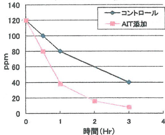
トリメチルアミンガス推移
